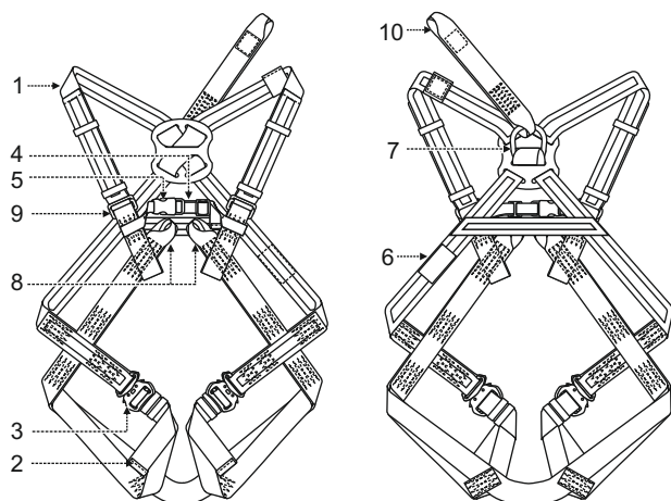
P-30EC / AB 130 02
