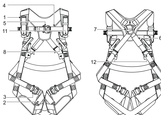
P-32PRO / AB 132 01
