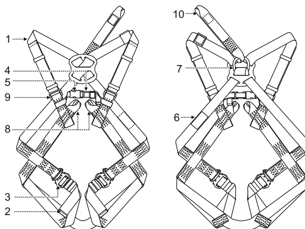
P-30C / AB 130 03
