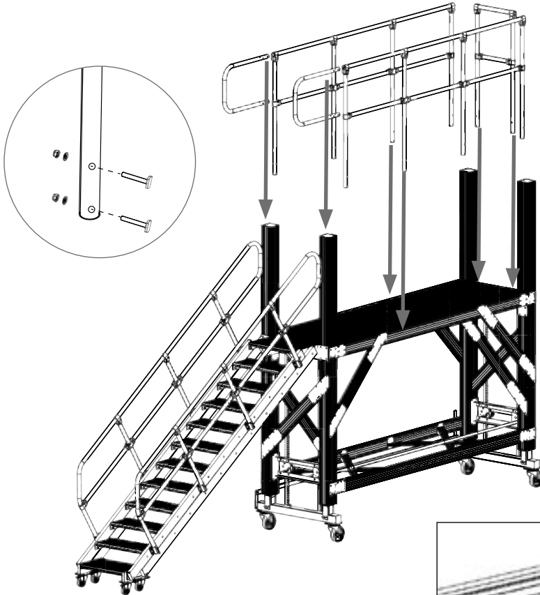
Kivehető korlát:
