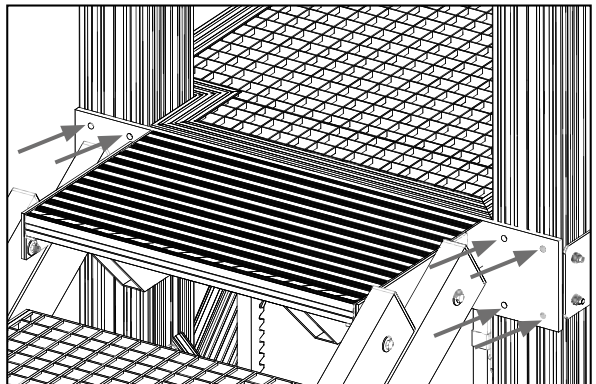
Detail:
