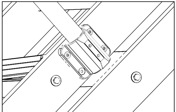
Detail Befestigung:
