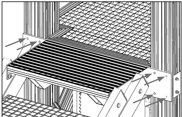
Detail:
