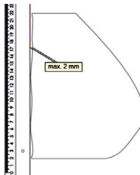
Rysunek 7. Szacowanie maksymalnej dopuszczalnej nierówności struktury betonowej
